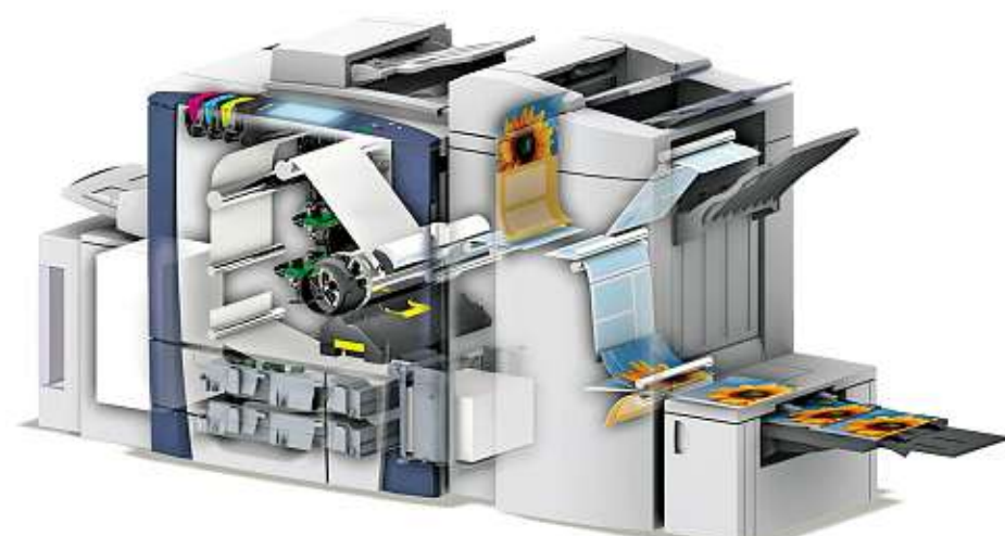
Tiskové zařízení Xerox ColorQube 9200 v částečném řezu.
